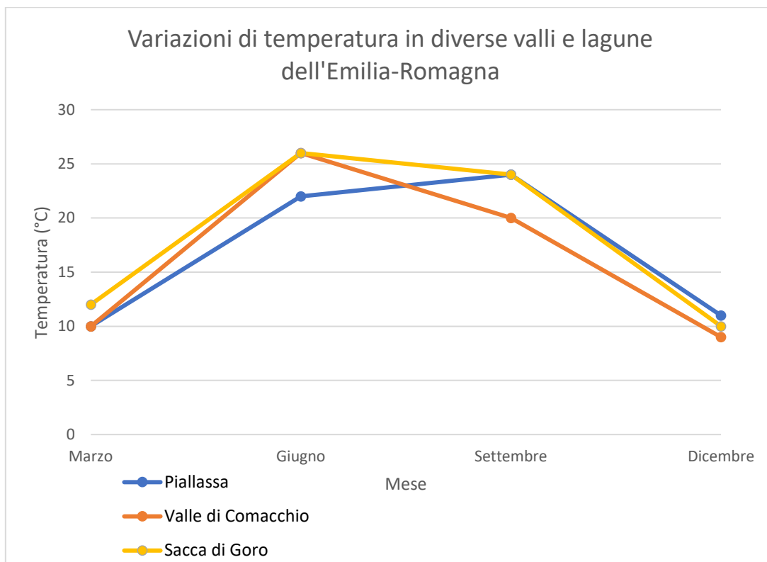
Grafico 4. Variazioni di temperatura in 3 siti in valli e lagune in Emilia-Romagna (Piallassa, Valle di Comacchio e Sacca di Goro) in 4 mensilità (Marzo, Giugno, Settembre e Dicembre) per valutare l'applicabilità in situ del progetto GO Restocking (dati: ARPAE)
